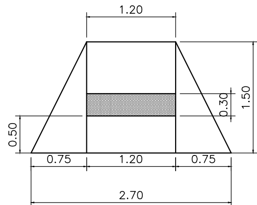
PLANTA ESQUEMÁTICA P/ RAMPAS DE ACESSIBILIDADE
