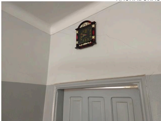
RACHADURAS 45° EM PAREDES
