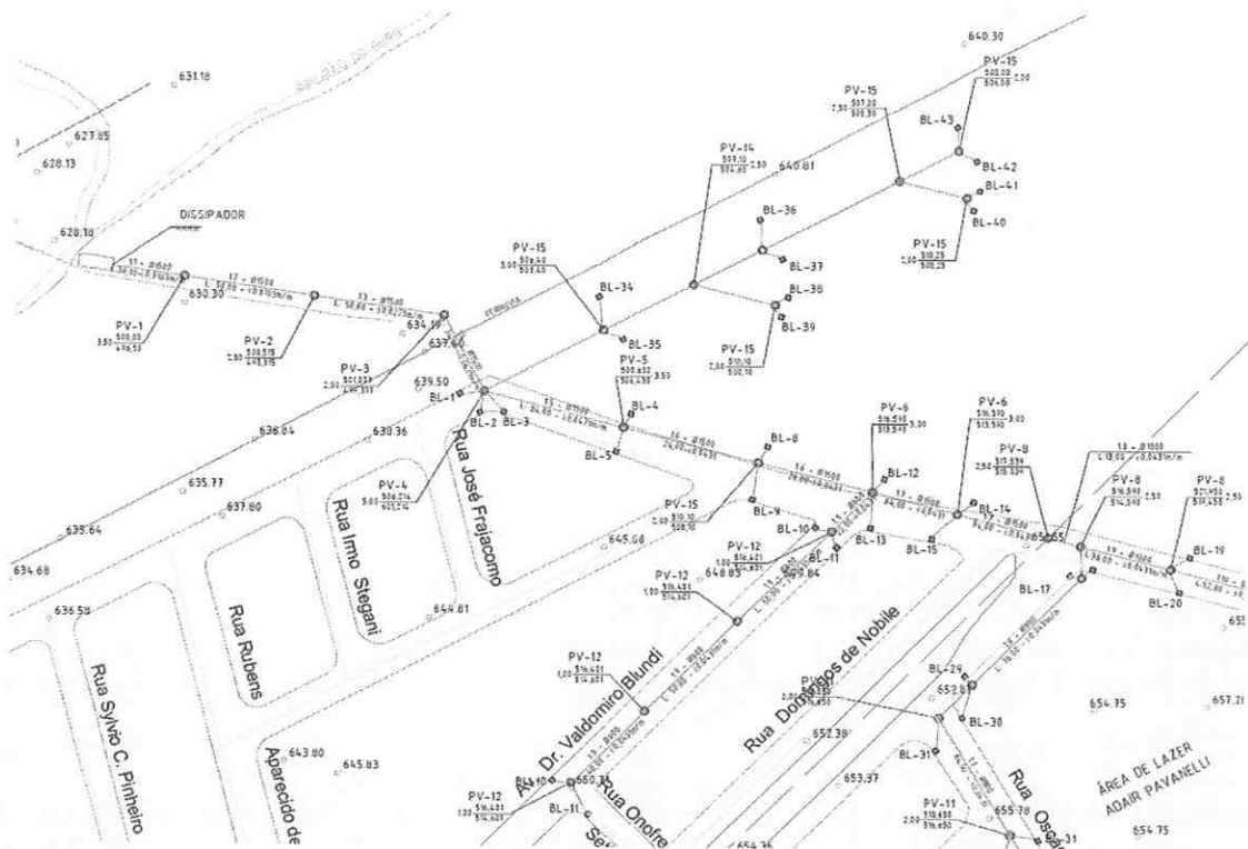
Imagem 1 – Traçado da rede projetada para o local, implantada até o limite da faixa de servidão da ferrovia
