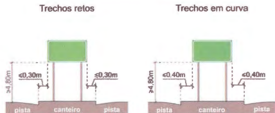
Figura 6 – Afastamento lateral e altura livre
