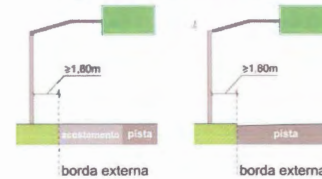
Figura 11 – Afastamento lateral
