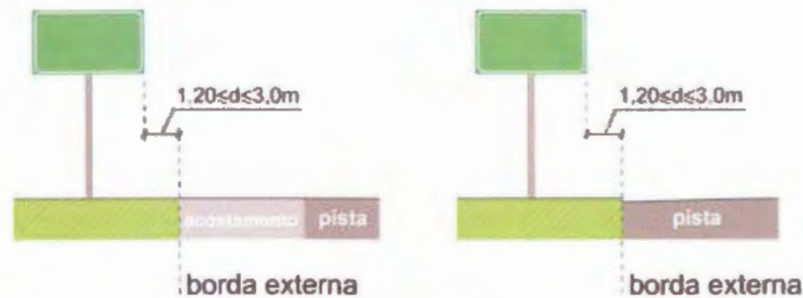
Figura 10 – Afastamento lateral
