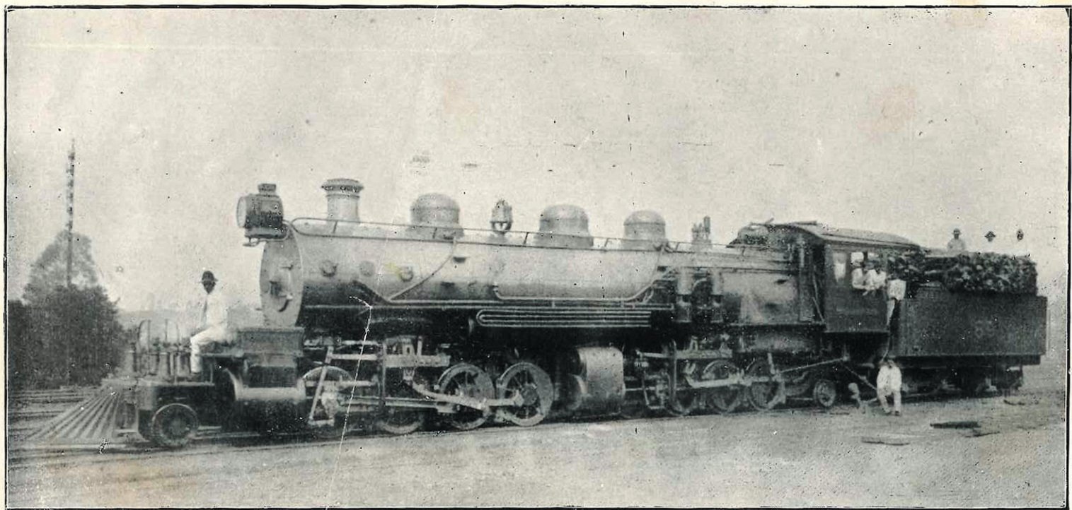
Locomotiva dupla (Malet), igual ao numero 90, as mais possantes que possui a Companhia para a bitola 1m,00, pucham 40 vagões carregados.
