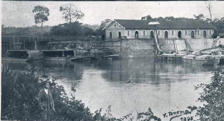
A nova ponte sobre o rio Mogy Guassú, em Porto Ferreira, que serve para o ramal de Santa Rita e estrada de rodagem Porto Ferreira, no tempo da Navegação Fluvial Paulista, vendo-se ao lado a antiga ponte de madeira.
