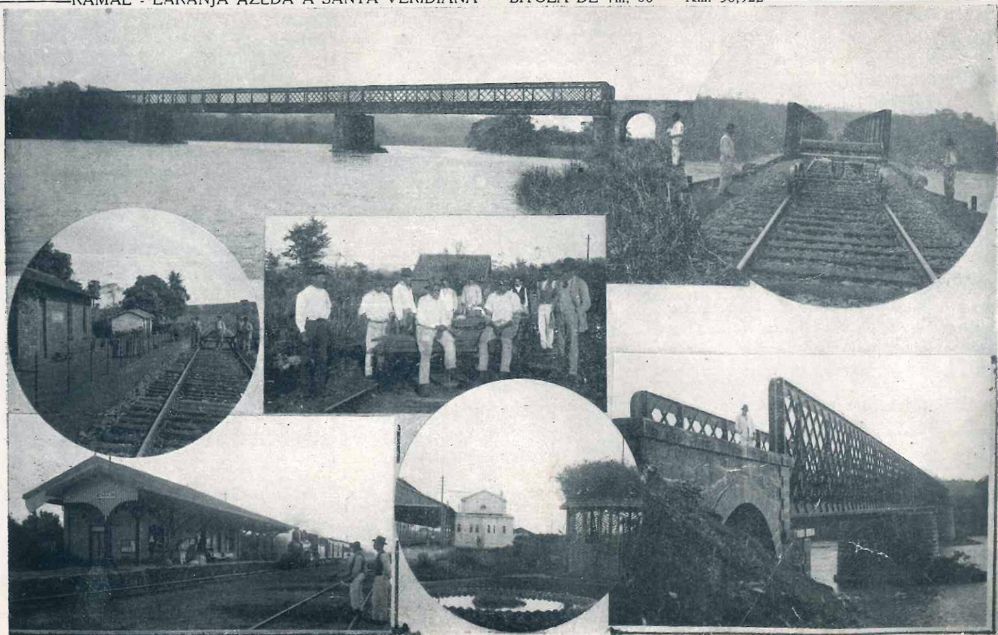
Ponte sobre o rio Mogy-Guassú no ramal de Santa Veridiana
